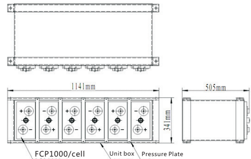
FCP-1000-12 module dimension
